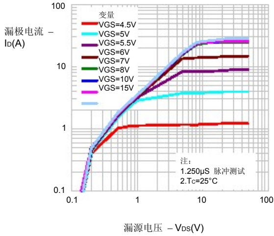
图1. 输出特性
