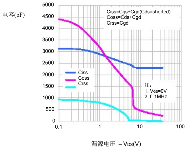
图5. 电容特性
