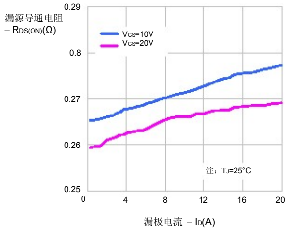
图3. 导通电阻vs.漏极电流、栅极电压
