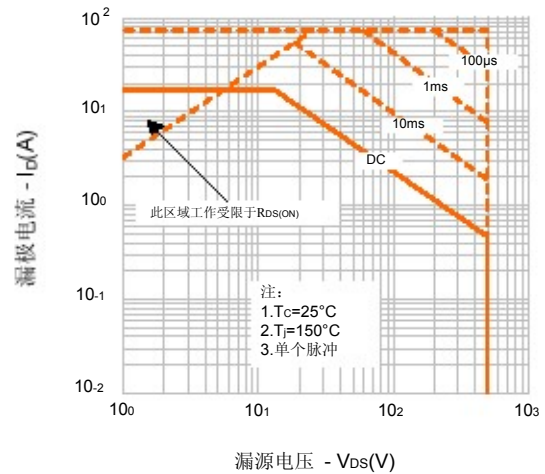
图9-2. 最大安全工作区域(SVF18N50PN)
