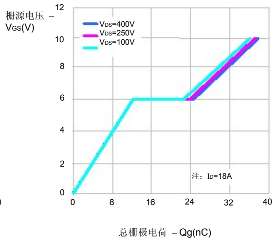
图6. 电荷量特性
