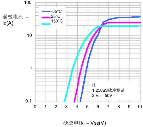
图2. 传输特性
